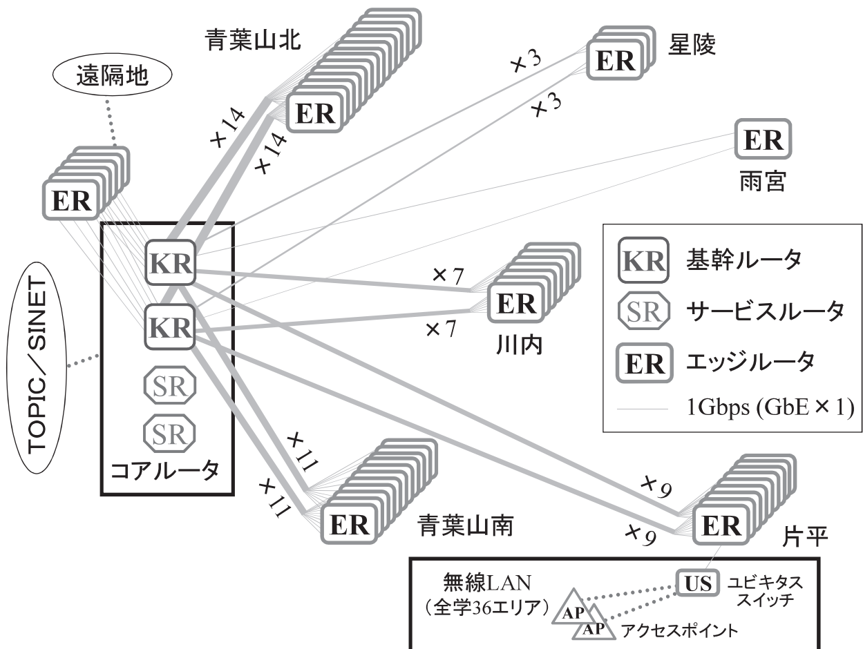
StarTAINS の構成
